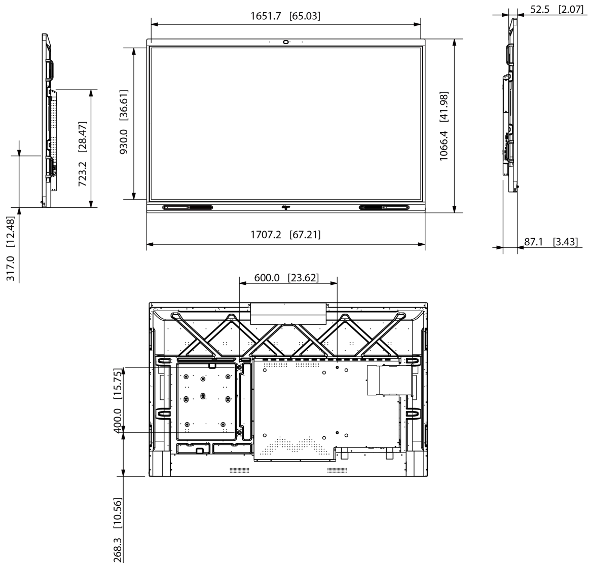
図1-3 寸法 (カメラ搭載機 : mm [インチ])
