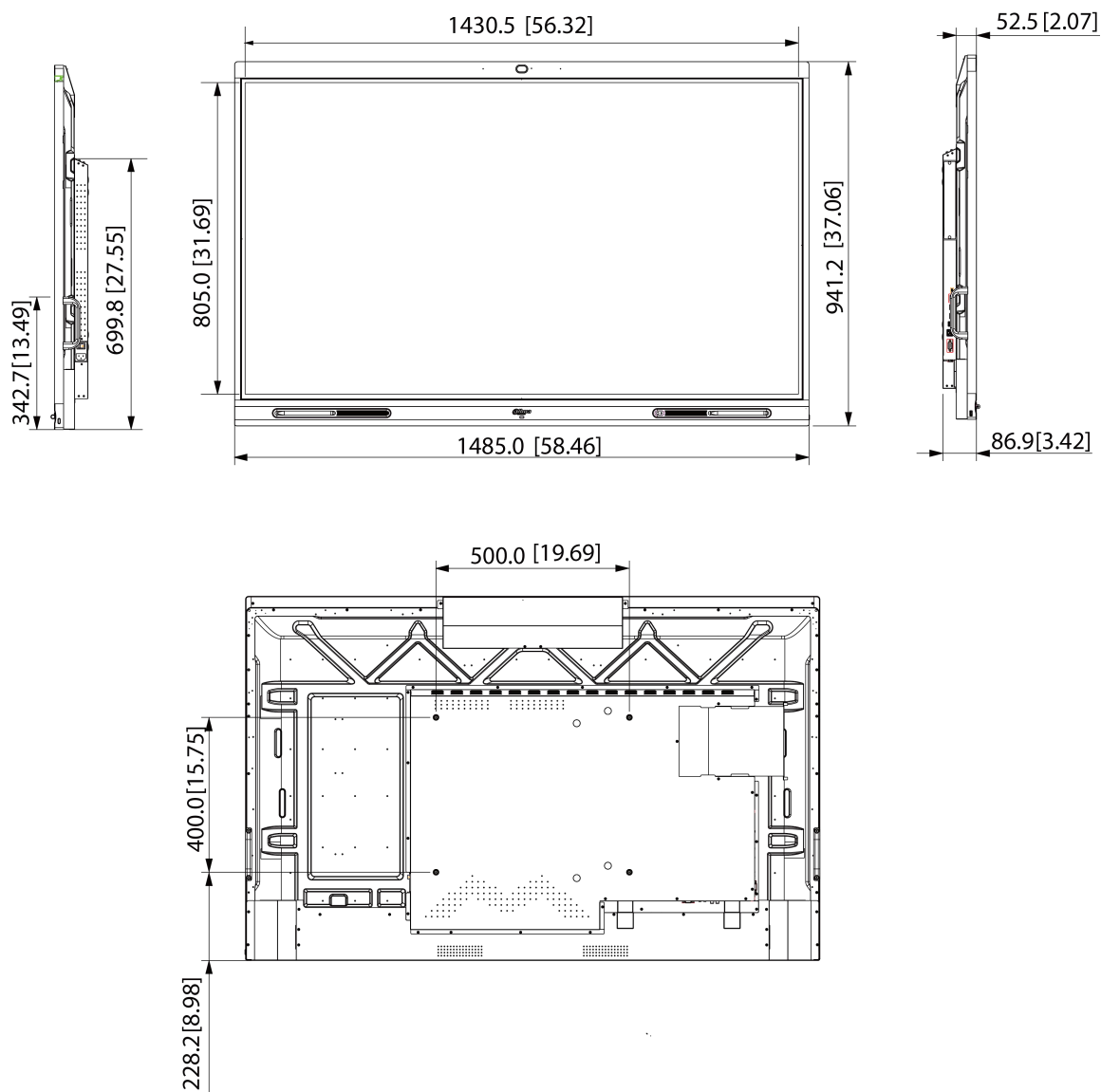
図1-2 寸法 (カメラ搭載機 : mm [インチ])
